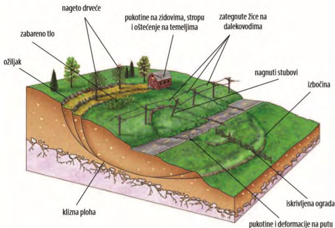
Slika 18: Prikaz pokazatelja nastanka klizanja
