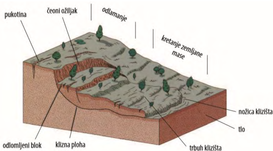
Slika 16: Prikaz osnovnih elemenata klizišta
