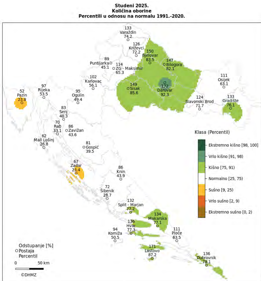
Slika 12: Prikaz odstupanja količine oborina u studenom 2025.god.
