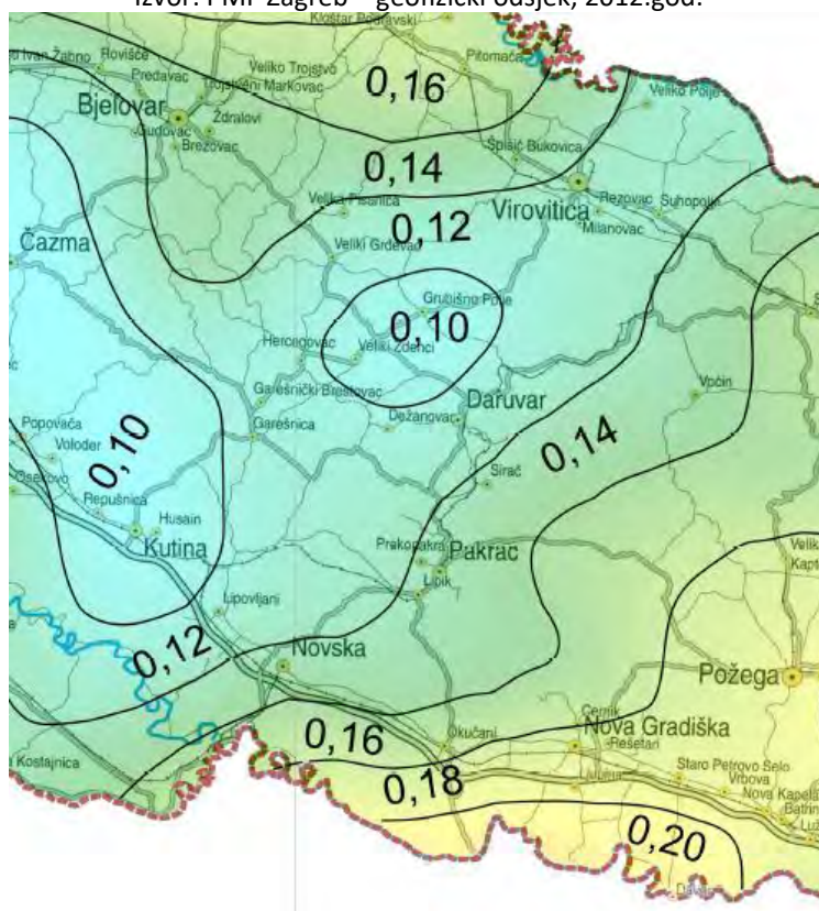
Slika 23: Karta potresnih područja za povratni period od 475 god. za dio Bjelovarsko - bilogorske županije Izvor: PMF Zagreb – geofizički odsjek, 2012.god.
