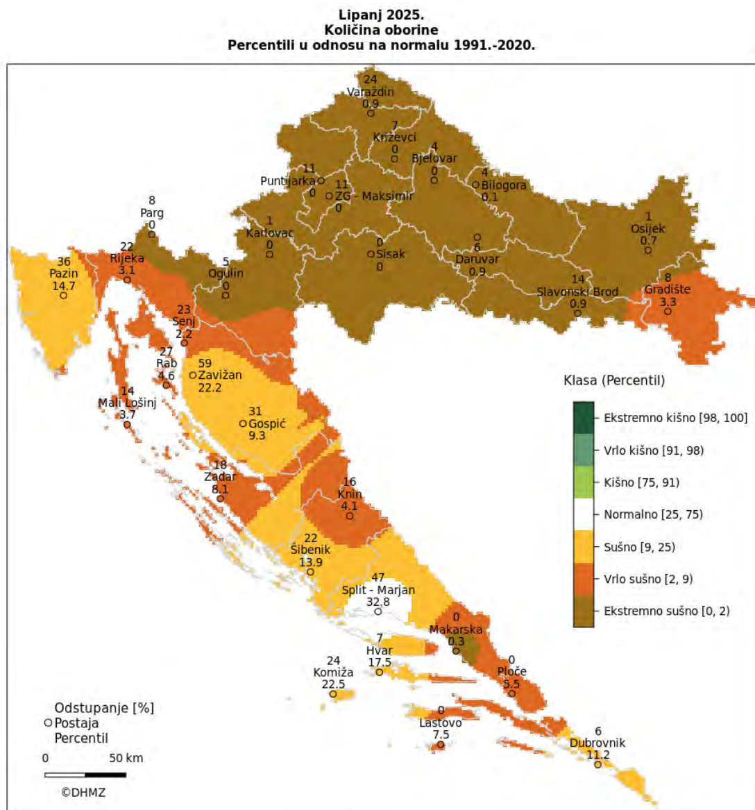
Slika 14: Prikaz odstupanja količine oborina za lipanj 2025.god.
