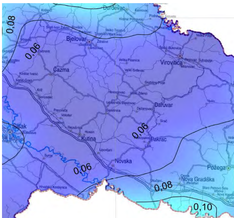
Slika 22: Karta potresnih područja za povratni period od 95 god. za dio Bjelovarsko - bilogorske županije Izvor: PMF Zagreb – geofizički odsjek, 2012.god.
